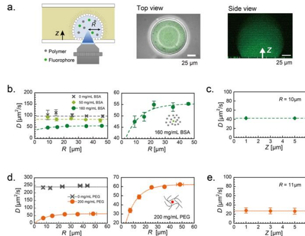
図 2. (a) 細胞モデル中での FCS 測定模式図 (左) 液滴を上から (中央) 側面から (右) 観察した図。(b) 様々な BSA 濃度における液滴サイズ R の GFP 拡散係数 D への依存性 (左) と、160 mg/mL BSA 溶液に対応する拡大図 (右)。(c) 160 mg/mL BSA-GFP 系での R = 10 \mu\text{m} 液滴中 D の z 位置依存性。(d-e) b, c に対応する実験の 200 mg/mL PEG を用いた結果。
