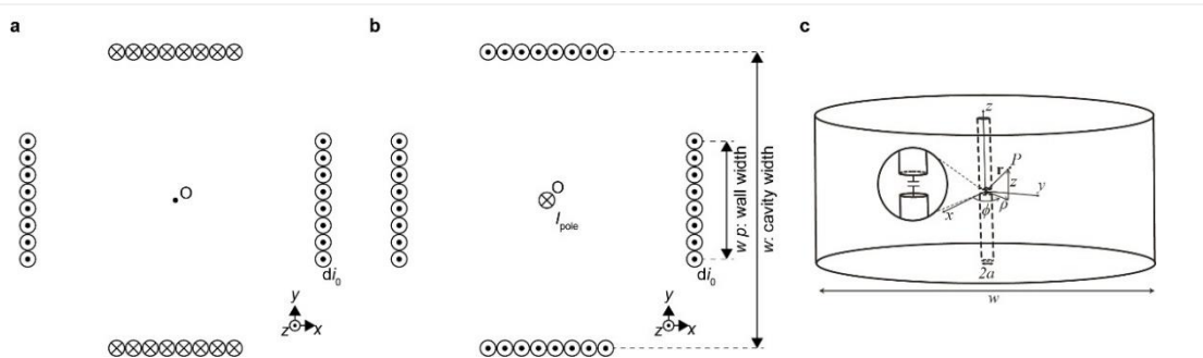
図 3 準静空洞共振器の磁界分布のモデリング方法の検討. (a, b) マルチモード準静空洞共振器の近似電流分布モデル. (c) 準静空洞共振器の解析に用いた近似構造.
