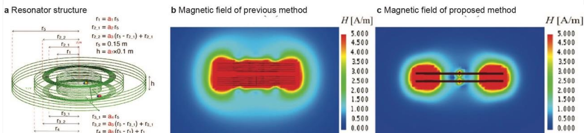
図 8 無線給電における漏洩磁界を抑制するためのハルバツハ配列共振器
