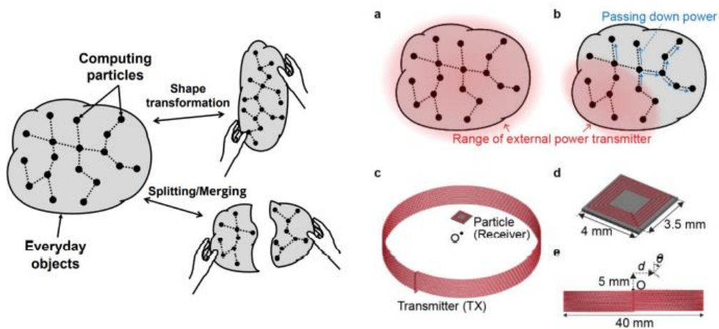
図 2 形状変化するコンピュータの無線ネットワーキングに向けた給電技術の検討。(a) 全体に対して送電器から電力を供給する方法と、(b) 一部の粒子にのみ電力を供給し、粒子間のネットワークにより電力を送り届ける方法。(c, d) 電磁界解析による粒子状のコンピュータへの無線電力伝送技術の検討。
