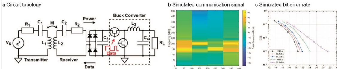
図 7 高効率な無線給電と通信の両立のための電力変換回路の変調による通信手法
