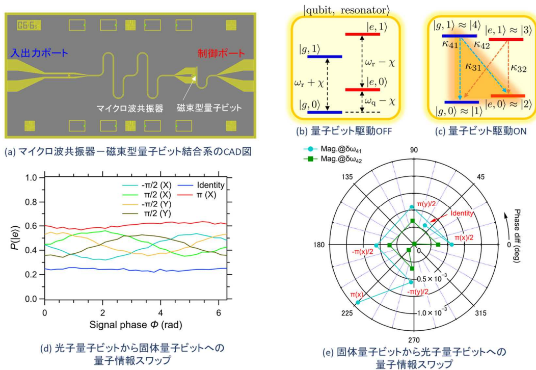
図1. 量子インターコネクションに向けた双方向量子メモリの実証
