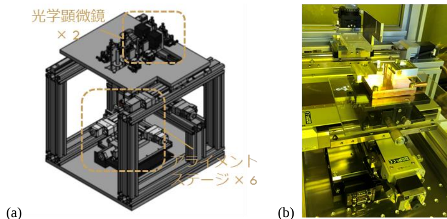
図 1 XFEL 計測用溶液試料ホルダ組立装置 (a) 装置の全体構成。 (b) 装置下部アライメントステージの拡大写真。
