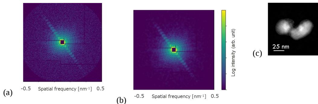
図 5 SACLA BL2 にて計測したナノ粒子からのコヒーレント回折パターンと再構成試料像。
