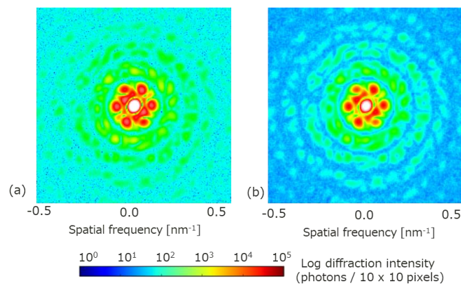
図 3 辞書学習を用いたコヒーレント回折パターンのノイズ除去シミュレーション。
