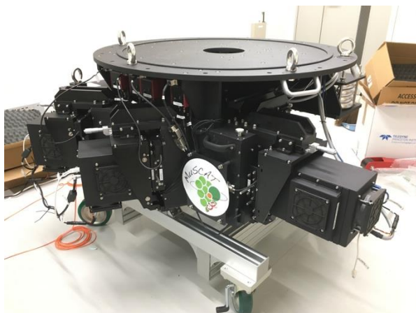
図 3: 左は東京大学で完成した MuSCAT3 の写真(2020 年 8 月)。右はマウイ島ハレアカラ山頂
