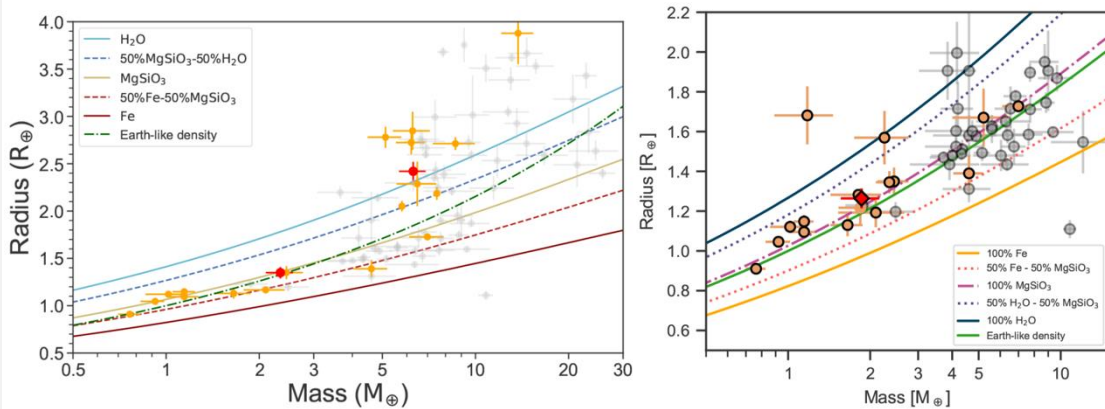
図 2: 左パネルの赤いデータは、MuSCAT2 で発見確認を行った 2 つの惑星 LTT 3780b と LTT 3780c(TOI732.01 と TOI732.02)の質量(横軸:地球質量単位)と半径(縦軸:地球半径単位)の関係(Nowak et al. 2020 の図 9 から引用)。橙色や灰色のデータは他の既知のトランジット惑星のデータ。実線や破線で示されているのは、惑星の組成を仮定した場合に理論的に予想される質量と半径の関係。緑色の破線が地球の組成を仮定した場合で、LTT 3780b が地球型惑星であることが示されています。同様に右のパネルの赤いデータは、MuSCAT と MuSCAT2 で発見確認を行った GJ 3473b(TOI488.01)の質量と半径の関係(Kemmer et al. 2020 の図 10 から引用)。こちらでは緑色の実線が地球の組成を仮定しており、この惑星も地球型惑星であることが示されています。これらの惑星は、将来の宇宙望遠鏡での惑星大気観測に適したターゲットであることがわかりました。
