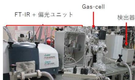
図 1. オペランド赤外分光装置写真
