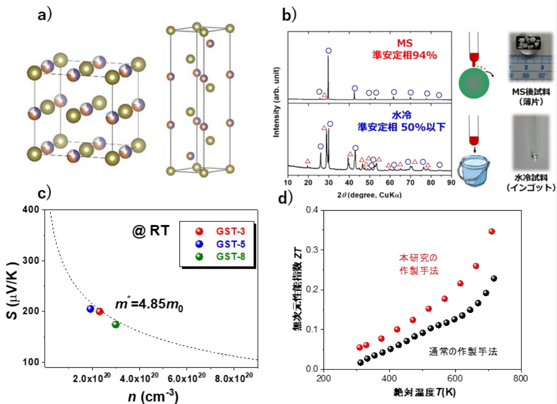
図3. a) 立方晶と六方晶の結晶構造。オリーブ色の球が Te 原子、青色/赤色/白色の原子が Ge/Sb/空孔で占められた原子を表す。 b)液体急冷凝固法(MS)と水冷で作製した試料の X 線回折パターン。MS 法で作製した試料では 90wt%以上の準安定相を含む試料が得られている事がわかる。c)液体急冷凝固法(MS)+室温高圧プレスで作製した試料のゼーベック係数 S のキャリア濃度 n 依存性。シングルパラボリックモデルで表せる事が示されている。d)相転移を利用した欠陥含有準安定構造の熱電特性。
