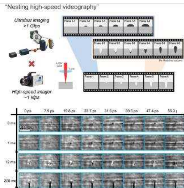
図2 入れ子型高速度イメージングの概念(上) と撮影例(下)
