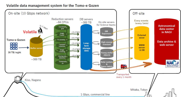
図 2. オンサイト逐次処理システムの概要
