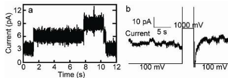
図 3 単一チャンネル電流測定(パッチクランプ測定)の一例と安定性の確認
