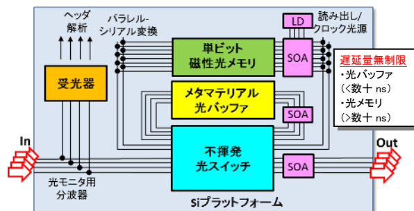
図 1.1: フォトニックルータの構成図
