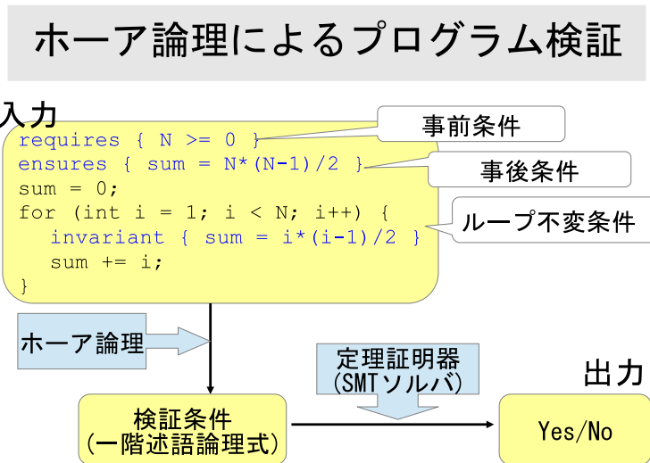
図 3.4.1 プログラム検証の流れ
