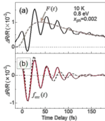
図 4.1-23 (a) 反射率変化の時間発展、(b) 振動成分 励起光中心エネルギー 0.8 \text{ eV} 、プローブエネルギー 0.8 \text{ eV}
