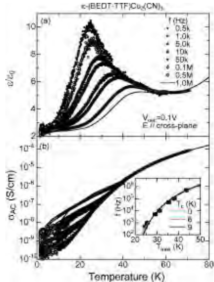
図 4.2-2 \kappa -(BEDT-TTF) 2 Cu 2 (CN) 3 の低周波誘電率に見られる異常なリラクサー的誘電分散[論文 2-6]
