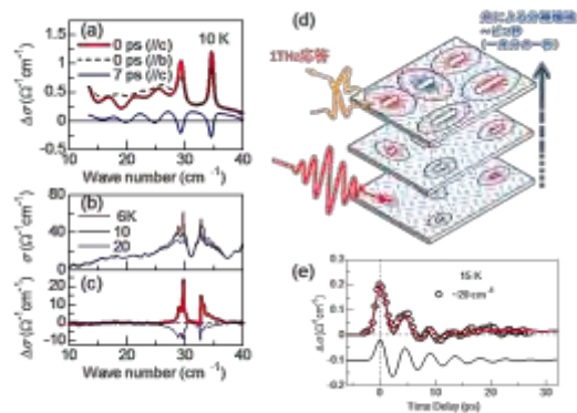
図 4.1-15 (a) 光励起 THz プローブ測定によって得られた光学伝導度の差分( \Delta\sigma )スペクトル。(b) 1THz のピークの温度依存性とその差分スペクトル。(c)
