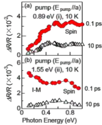
図 4.1-22 (a) 0.89 \text{ eV} および (b) 1.55 \text{ eV} の励起光照射後に観測される過渡反射スペクトル
