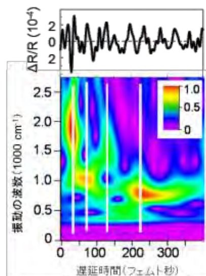
図 4.1-6 反射率変化の振動成分のスペクトログラムと、そのスペクトログラム (振動数の時間変化)
