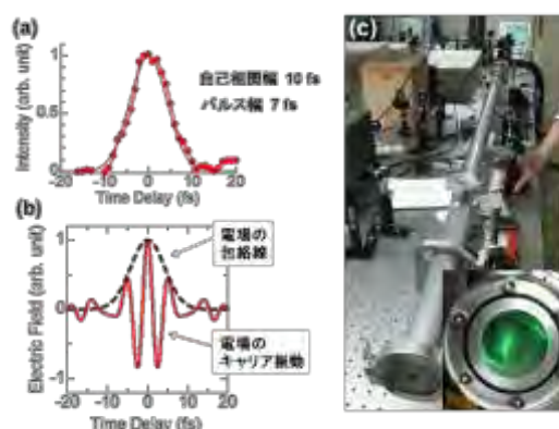
図 4.1-4 (a)自己相関関数と、(b)スペクトルのフーリエ成分として得られる電場波形 (c)Kr 封入中空ファイバーシステムの概観
