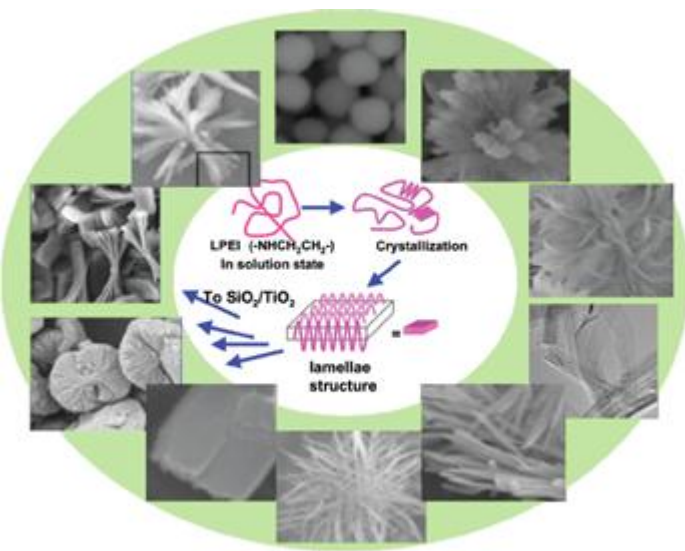
図 25 LPEI 結晶体から誘導されるシリカ/酸化チタンナノ構造体
