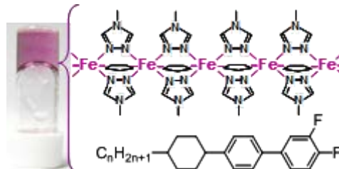
図 3 一次元 Fe II ( 1 ) 3 Cl 2 錯体による LS 液晶ゲルの形成 A-29)
