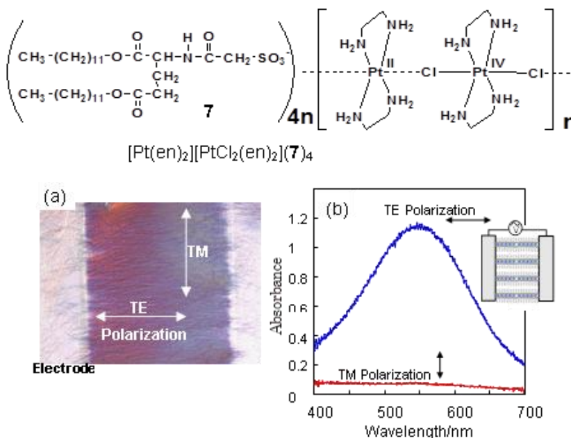
図 24 (a)電極間に配向した [Pt(en)_2][PtCl_2(en)_2](7)_4 錯体ナノファイバーの光学顕微鏡像、(b)偏光スペクトル
