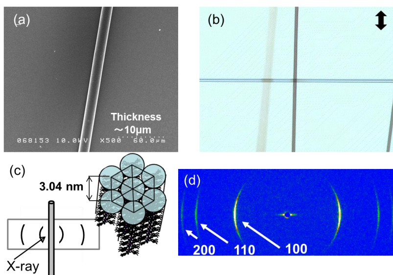
図 5 (a)ハロゲン架橋金属錯体 \mathbf{3} ( X = \text{Cl} ) \mu ファイバーの SEM 像 (b)偏光顕微鏡写真(二本の \mu ファイバーが直交) (c) \mu ファイバーの小角X線測定(SAXS)模式図 (d) \mu ファイバーの小角X線回折像
