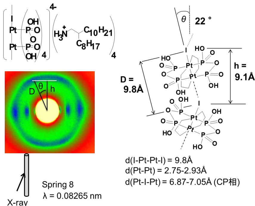
図6 ハロゲン架橋金属錯体 4 の構造ならびに \mu ファイバーの小角X線回折像(Spring 8), 一次元鎖のジグザグ構造モデル
