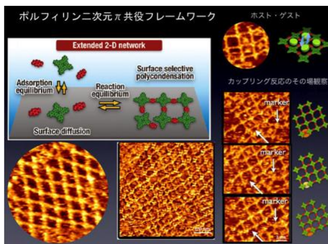
図 18 ポルフィリン二次元 \pi 共役フレームワークの STM その場観察 A-22)
