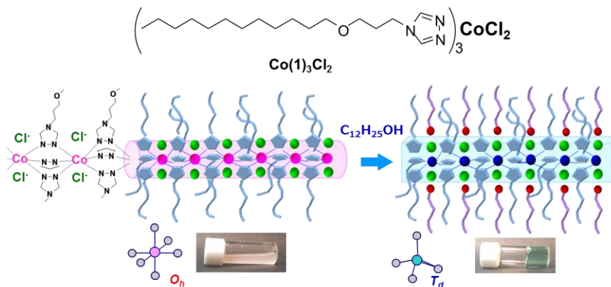
図1 一次元 \text{Co}^{\text{II}}(\mathbf{1})_3\text{Cl}_2 錯体表面へのゲスト結合により誘起される配位構造変化の模式図 A-40)
