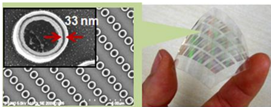
図 23 ポリマーフィルム上に作製した金二重ナノピラー配列 作製したギャップ幅 33 ナノメートルの金二重ナノピラーの電子顕微鏡写真(左)とそれらを配列させたポリマー基板の全体像(右)
