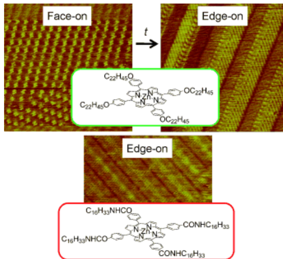
図 20 固-液界面における長鎖 Zn(II) ポルフィリンの二次元組織化制御 C-2)
