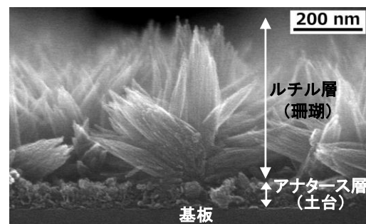
図 26 \text{TiO}_2 ナノコーラルの断面 SEM 写真 A-9)
