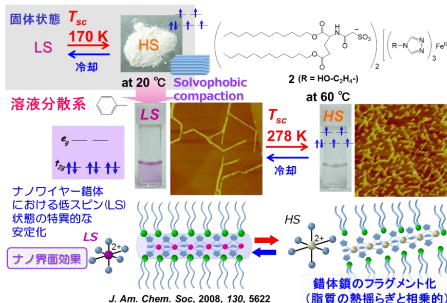
図2 ナノワイヤー \text{Fe}(\text{II}) 錯体における“ナノ界面効果”と spin conversion 現象 A-38)
