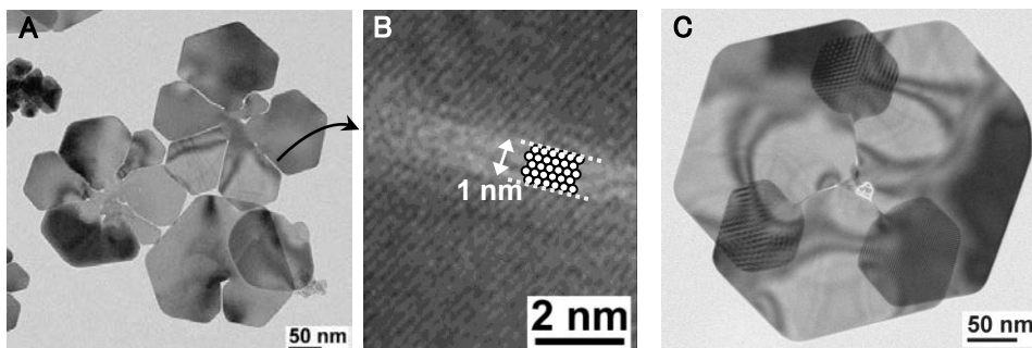
図 14 ナノ彫刻法により得られた花冠状金ナノプレート単結晶の TEM 写真 A-31)
