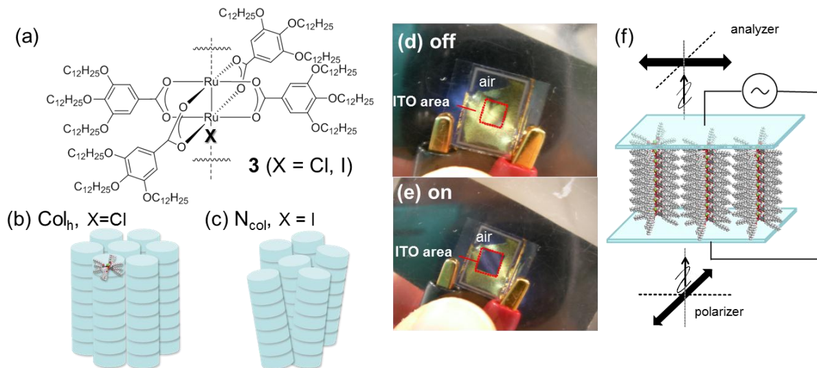
図 4 (a) 脂溶性 MMX 型ハロゲン架橋金属錯体 \mathbf{3} ( X = \text{Cl}, \text{I} ) (b)ヘキサゴナルカラムナー( \text{Col}_h )相 ( X = \text{Cl} ), (c)カラムナーネマチック( \text{N}_{\text{Col}} )相( X = \text{I} ), (d,e) \mathbf{3} ( X = \text{Cl} )デカン溶液を ITO 電極に挟んだ試料の写真(クロスニコル下)(d)交流電場無印加時 (e)交流電場( 0.8 \text{ V } \mu\text{m}^{-1} , 100\text{Hz} )印加時。赤枠線内は ITO 電極部位。(f)交流電場印加時における \mathbf{3} ( X = \text{Cl} )の誘電配向模式図 A-11)
