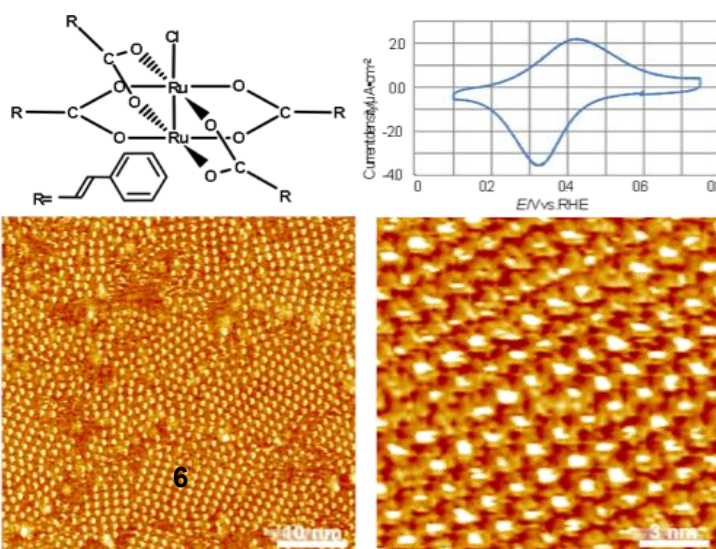
図 16 二次元配列した MMX 型錯体 6 の高解像度電気化学STM像とサイクリックボルタモグラムの A-5)
