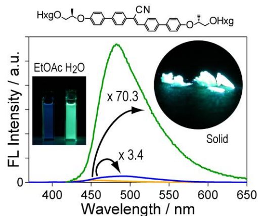
図 21 1-シアノ 1,2-ビスビフェニル エテン誘導体の AIEE 特性 C-7)
