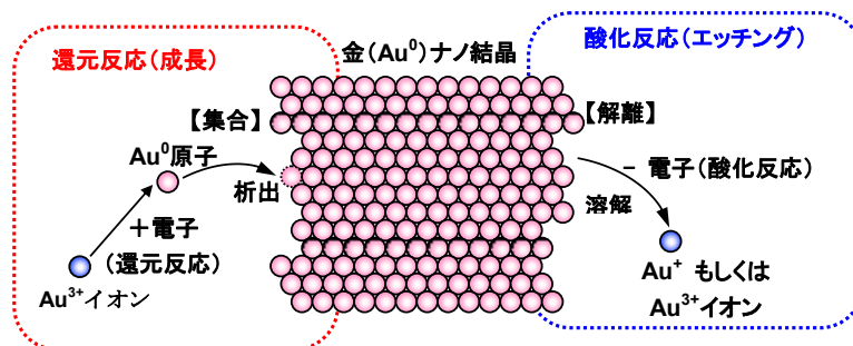
図 13 ナノ彫刻法概念。 A-31 Au 3+ の還元反応による Au 結晶の生長と酸化溶解反応(エッチング)を共存させ、化学反応を伴いながら原子が集合—解離する“自己組織化”プロセスを実現することによって、動的なナノ界面構造が生み出される。
