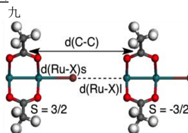
図 22 1次元 RuRuX 鎖の計算に用いたユニットセル.
