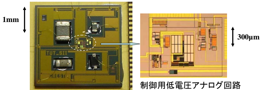
図6 CMOS 上に SMD を一体化した無線発電機構の試作チップ写真
