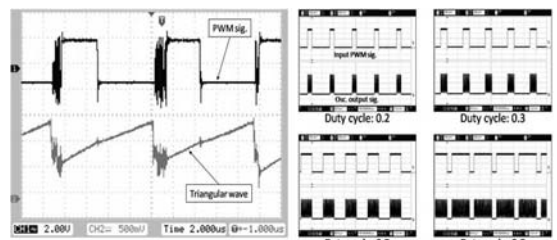
三角波・パルス幅変調波の出力 異なるパルス幅信号によるVCOの出力
