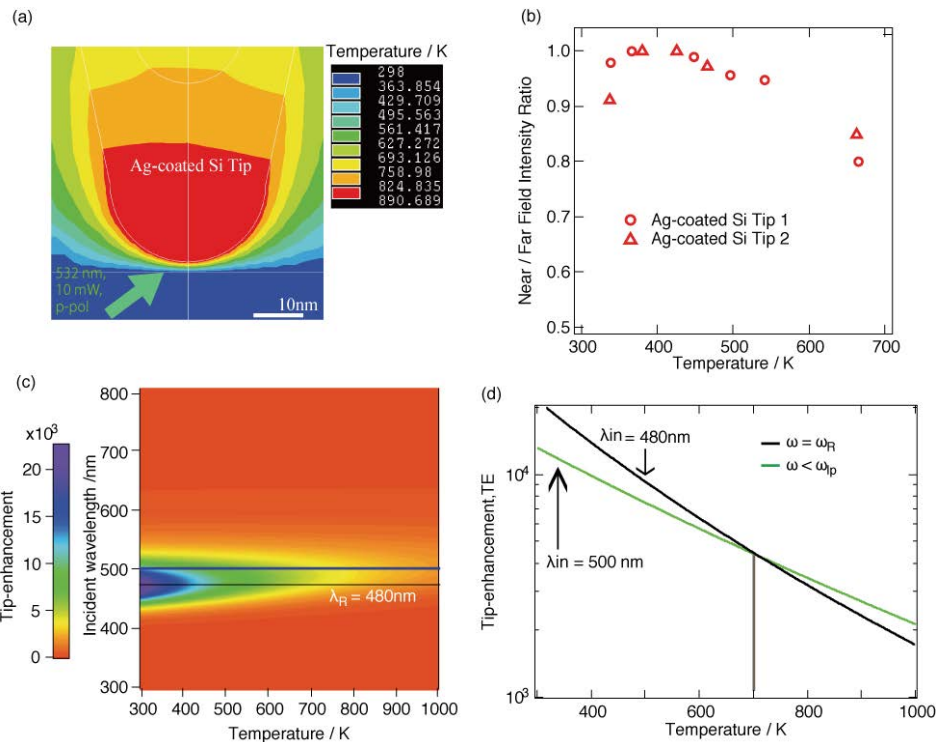
図 1 3 (a) レーザー照射時の銀ナノ探針先端の温度分布 (有限要素法計算結果)。 (b) ラマン散乱光増強度の探針温度依存性。 (c) SPP共鳴スペクトルの温度依存性 (電磁場計算結果)。 (d) 入射光波長が480nmおよび500nmの時の電場増強度の温度依存性。
