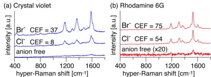
図8 ハロゲン化物イオン (Br - , Cl - ) を添加したときの色素分子の表面増強ハイパーラマン散乱スペクトルと、それぞれの化学増強度(CEF)。(a) クリスタルバイオレット。(b) ローダミン 6G。
