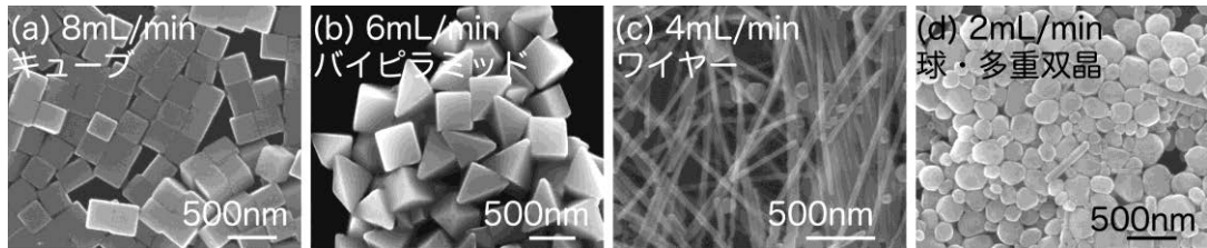
図7 酸素流量により形状制御された銀ナノ結晶のSEM像。酸素流量を(a) 8mL/min、(b) 6mL/min、(c) 4mL/min、(d) 2mL/min に制御して合成した結果、それぞれ(a) キューブ、(b) バイピラミッド、(c) ワイヤ、(d) 球および多重双晶が高収率で得られた。
