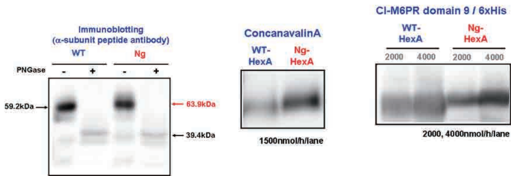
図4 N-グリカン付加配列追加によるヒト Ng-HexA への M6P 含有型糖鎖の追加
