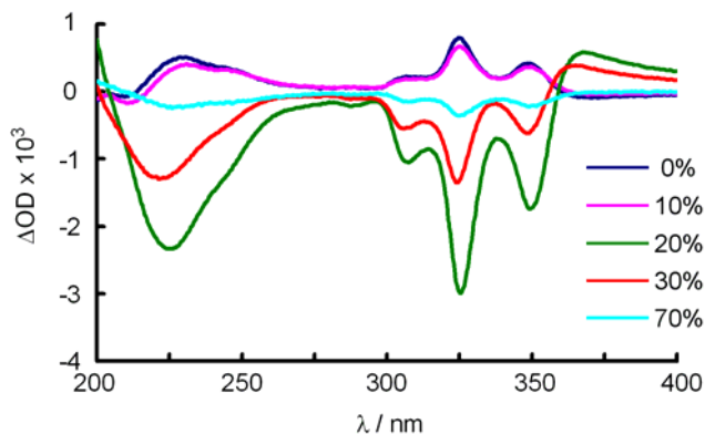
図2-2.マクロサイクル( S )-8cの固体薄膜の誘起CDスペクトル(CH 3 OH in CHCl 3 = 0-70%, 3.8 × 10 -3 M)
