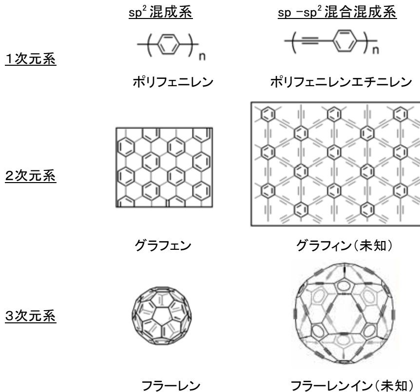
図1. 1次元、2次元、3次元構造を有する sp^2 混成および sp-sp^2 混合混成パイ電子系
