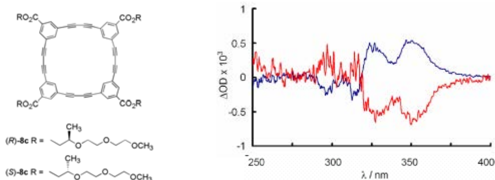
図2-3.マクロサイクル( R )-8c(赤) ( S )-8c(青)の溶液中の誘起CDスペクトル(CH 3 OH/CHCl 3 = 8/2, 2.5 × 10 -4 M)
