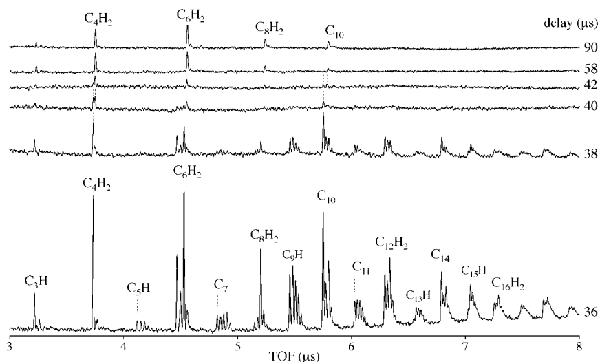
図 3-10 . 炭素棒のレーザー蒸発により H_2 中で生成する分子の 1 光子イオン化質量スペクトル
