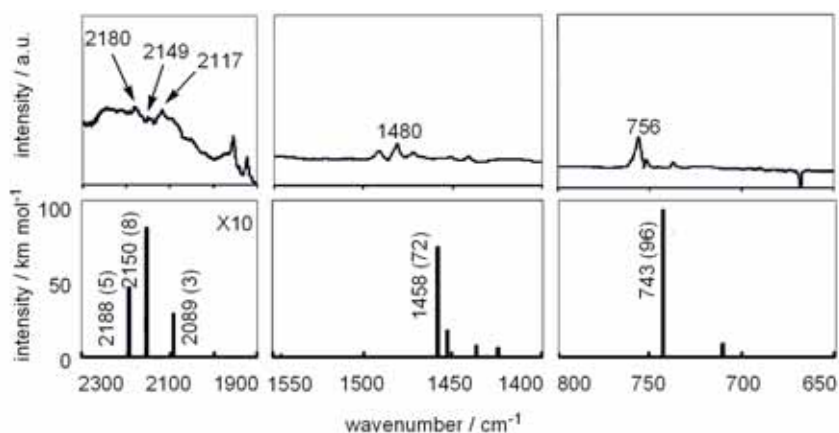
図 3-2 . (上段) アルゴン中 20 K 下で前駆体 2 を照射して得られた FT-IR 差スペクトル (下段) DFT 計算(B3LYP/6-31G*)に基づく 1 の理論 IR スペクトル
