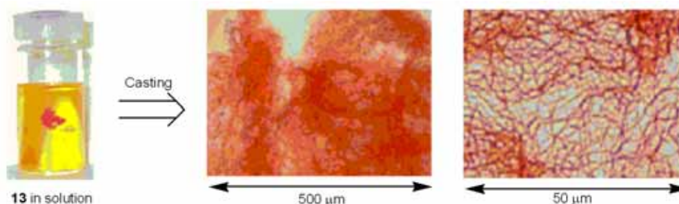
図 2-10 . 巨大環状分子 13 から得られた分子ワイヤー
