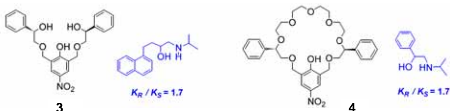
図1-3 .ポダンド型ホスト分子3および24-クラウン-8型ホスト分子4とそれぞれのキラル第二級アミンに対する不斉選択性の例
