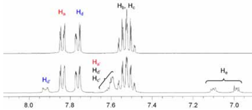
図 3-3 .(上段) 前駆体 6 の ^1\text{H} NMR スペクトル (THF- d_6 ) (下段) 光照射後の ^1\text{H} NMR スペクトル . 5 とインダンのシグナルが観測される .
