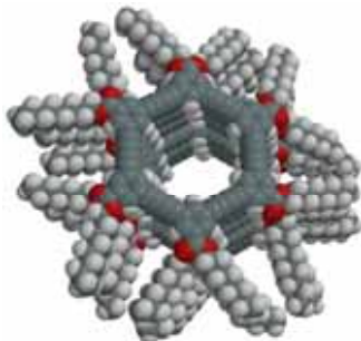
図 2-1 . ナノチューブ状構造を持つマクロサイクルの 1 次元会合体
