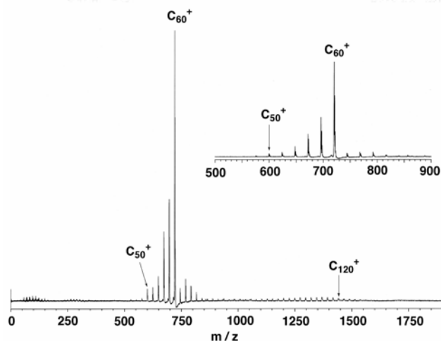
図 3-5 C_{60} 前駆体 8b の陽イオンモード LD TOF マスペクトル。(挿入) C_{60} 付近の拡大
