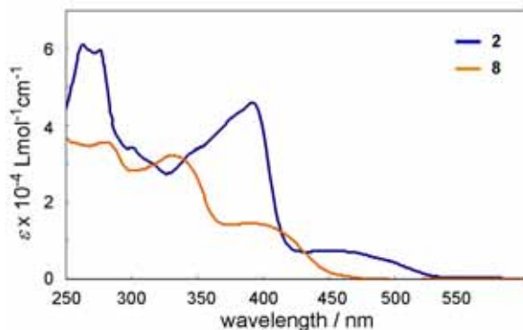
図 2-11 . 化合物 2 (青) と 8 (赤) の THF 中における UV-vis スペクトル
