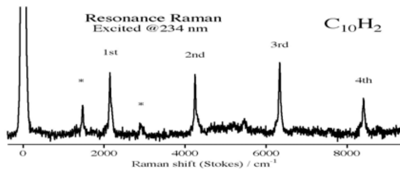
図 3-9 . ポリイン分子 C_{10}H_2 の共鳴ラマンスペクトル (ヘキサン溶液)
