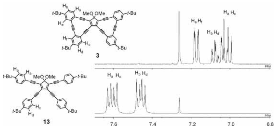
図 2-13 . 化合物 3 と 13 の ^1\text{H} NMR スペクトル ( \text{CDCl}_3 )
