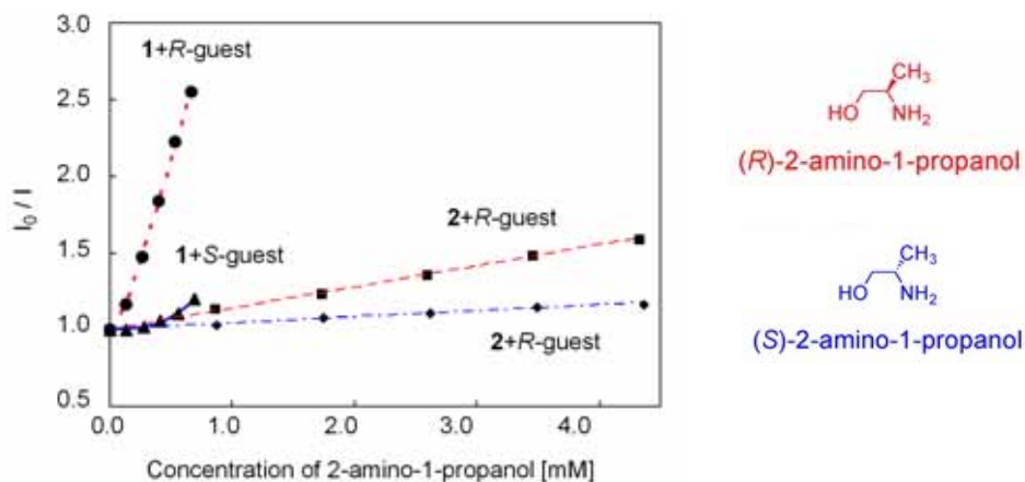
図 1-1 . PPE 1 とモデル分子 2 の蛍光消光の Stern-Volmer プロット
