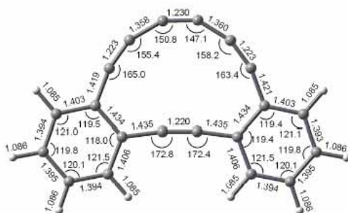
図 3-1 . 高ひずみ[12]DBA 1 の DFT 計算 (B3LYP/6-31G * ) による理論的構造
