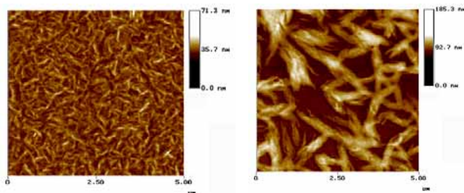
図 2-4 .マクロサイクル( S )-8c を石英基板上にスピコートして得られた薄膜の AFM 像 .(左) \text{CHCl}_3 (右) \text{CH}_3\text{OH}/\text{CHCl}_3 = 2/8
