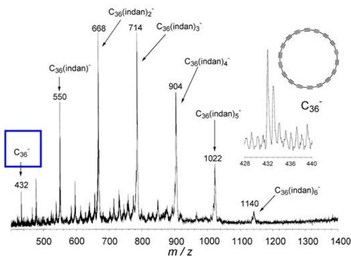
図 3-4 .ラジアレン型シクロカーボン前駆体 7d の LDMS マスペクトル
