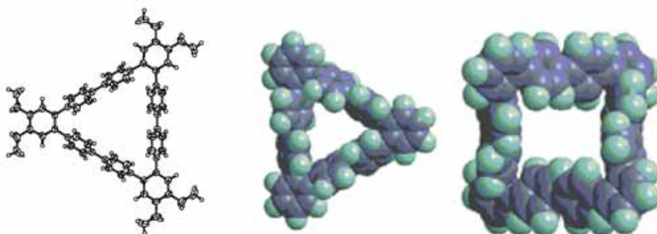
図 4-4 .(左) ノナフェニレン 19b の X 線結晶構造 .(中) ノナフェニレン 19a の理論的構造(HF/6-31G * ) .(右) ドデカフェニレン 20a の理論的構造(HF/6-31G * ) .
