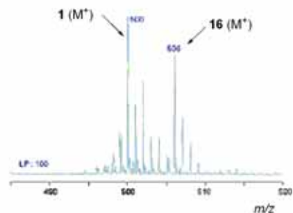
図 4-3 . 不飽和シクロファン 16 の LD TOF マススペクトル . シクロフェナセン 1 ( m/z = 500 )の生成が観測された .
