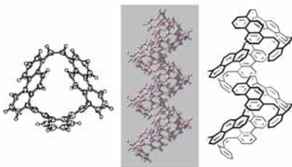
図 4-2 .不飽和シクロファン 16 のX線結晶構造とそのパッキング
