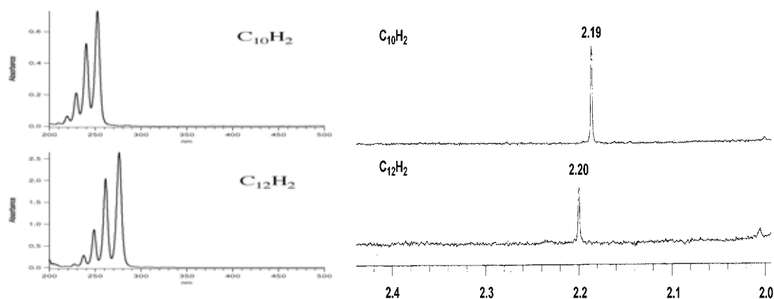
図 3-8 . (左) 直鎖ポリイン分子の UV 吸収スペクトル . (右) ^1H -NMR スペクトル .
