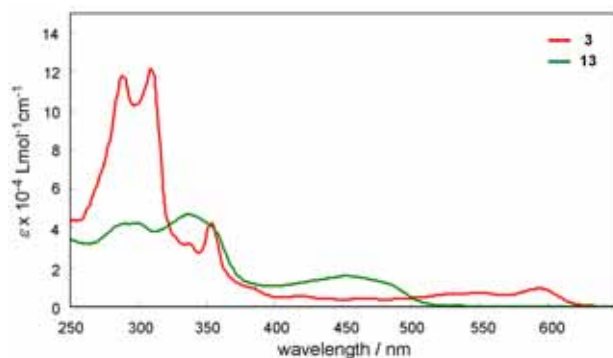
図 2-14 . 化合物 3 (赤) と 13 (緑) の THF 中における UV-vis スペクトル
