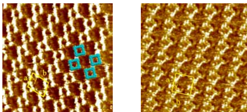
図 2-5 . マクロサイクルの HOPG/TCB 界面における 2 次元結晶の STM 像 .(左) ピリジノファン 10 (青色は 10 の分子模型)(右) シクロファン 8a
