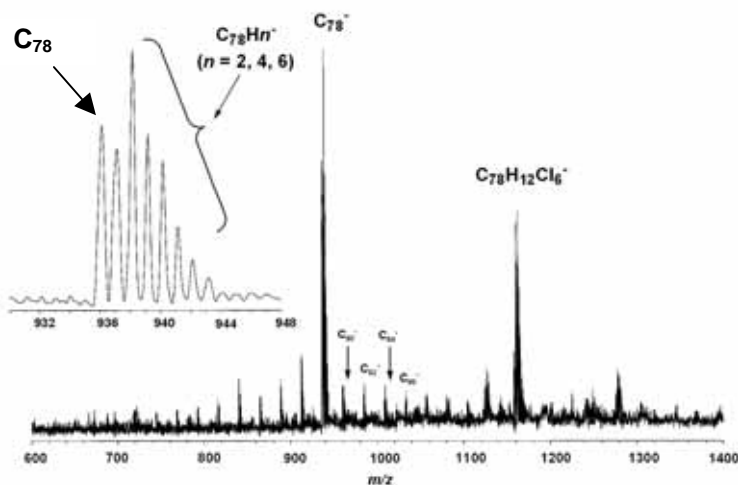
図 3-7. C_{78} 前駆体 12b の陰イオンモード LD TOF マススペクトル。(挿入) C_{78} 付近の拡大
