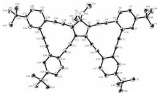
図 2-12 . バタフライ型 2 縮環式化合物 3 の X 線分子構造
