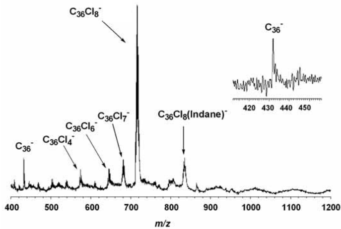
図 3-6 . C_{36} 前駆体 10b の陰イオンモード LD TOF マスペクトル .(挿入) C_{36} 付近の拡大
