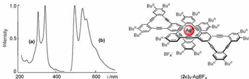
図 2-8 . (a)化合物 2 の電子スペクトルと (b) 蛍光スペクトル
