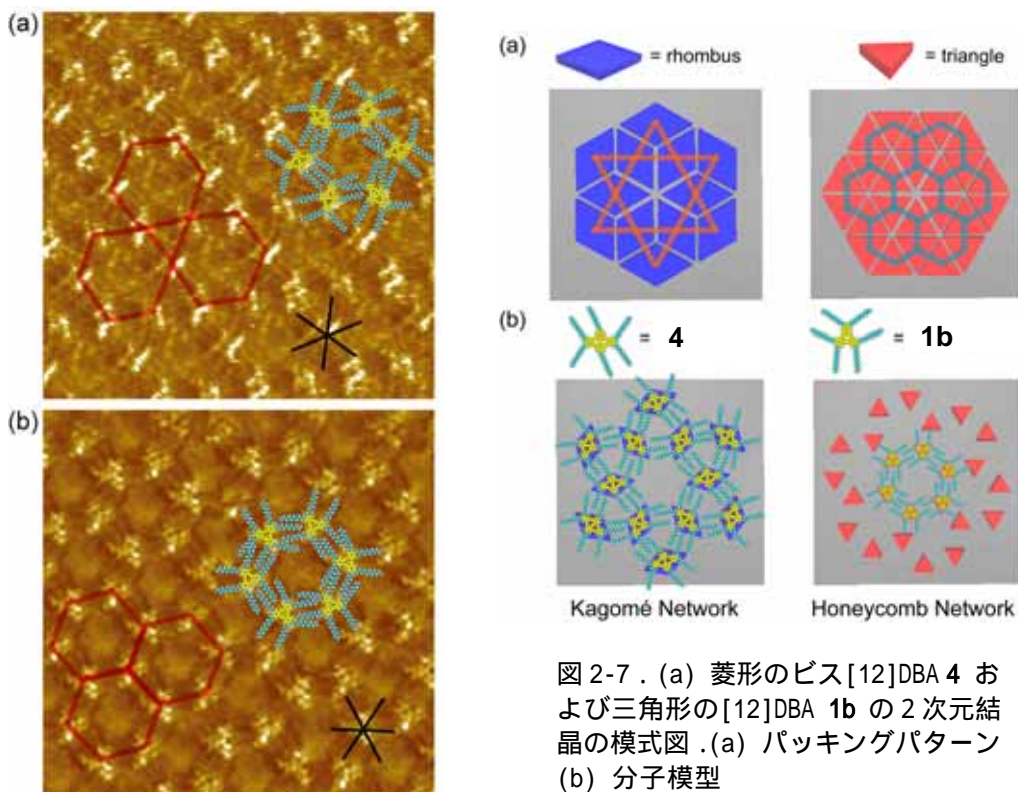
図 2-6 . デヒドロベンゾアヌレン類の固(HOPG)/液(TCB)界面における2次元結晶のSTM像 . (a) 菱形のビス[12]DBA 4 (b) 三角形の[12]DBA 1b
