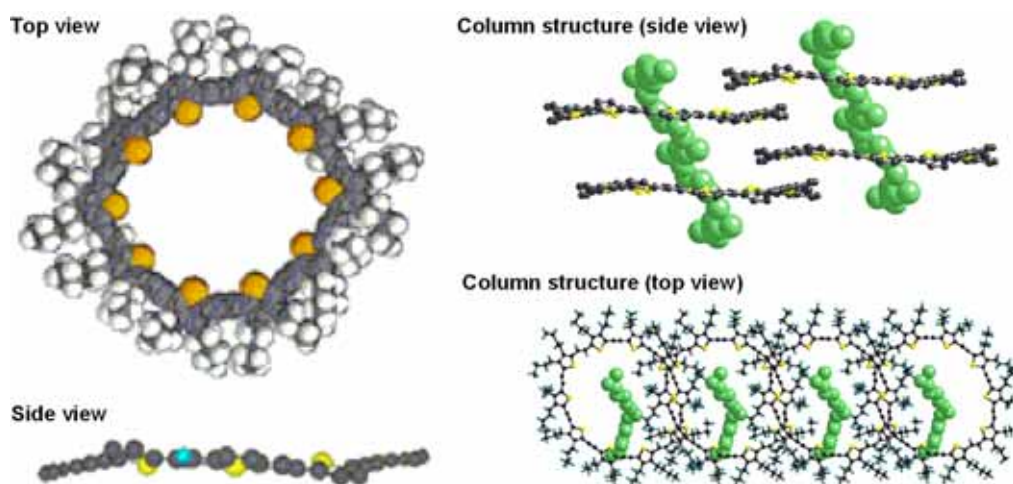
図 2-9 . 巨大環状分子 11 の X 線結晶構造解析
