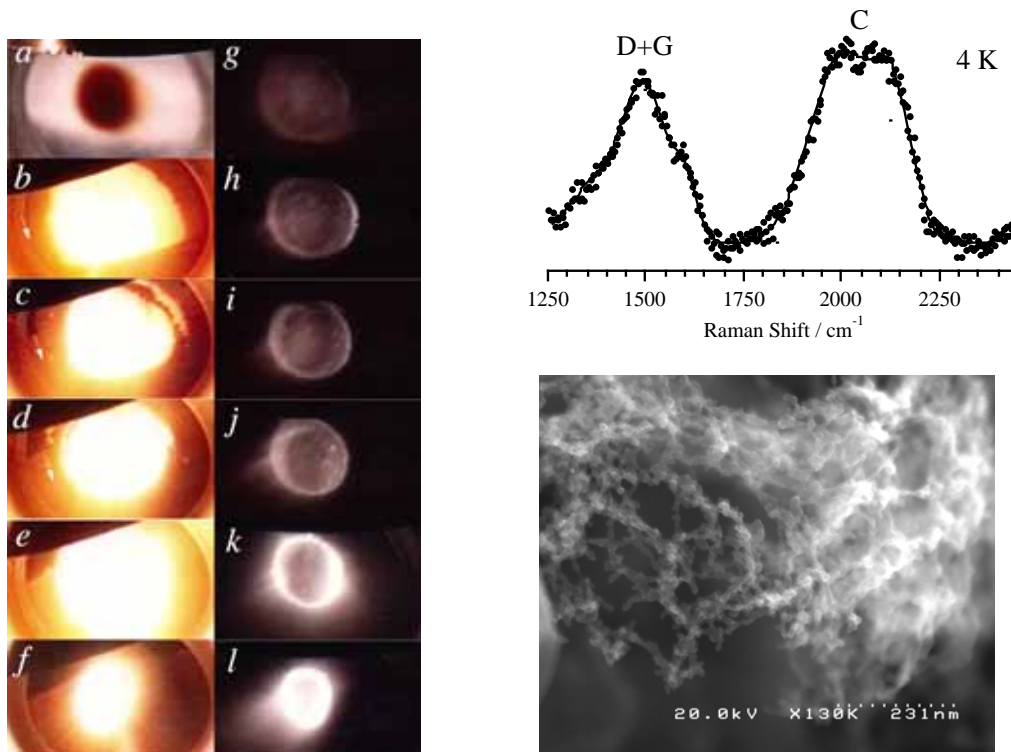
図 3-11 .(左) アルゴンマトリックス中での鎖状炭素クラスターの発熱的重合反応 . a. アニール前 b-f. アニール後、閃光を放ちながら重合が起こる様子 . g-l. 数回の反応の後、反応が終息していく様子 .(右 上)凝集体のラマンスペクトル .(右下)凝集体の電子顕微鏡像 (FE-SEM) .
