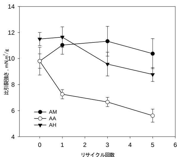
図9 リサイクル回数とアカシア材パルプ繊維シートの引張強さ
