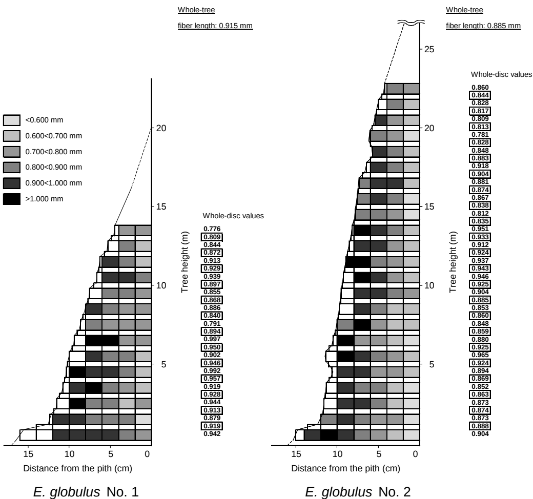
図 18 E. globulus における繊維長の樹幹内変異
