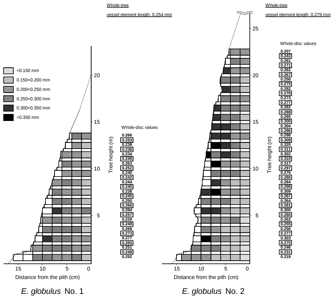
図 12 E. globulus における道管要素長の樹幹内変異
