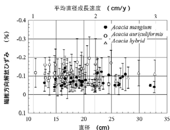
図 34 アカシア類の成長応力解放ひずみと平均直径成長速度の関係
