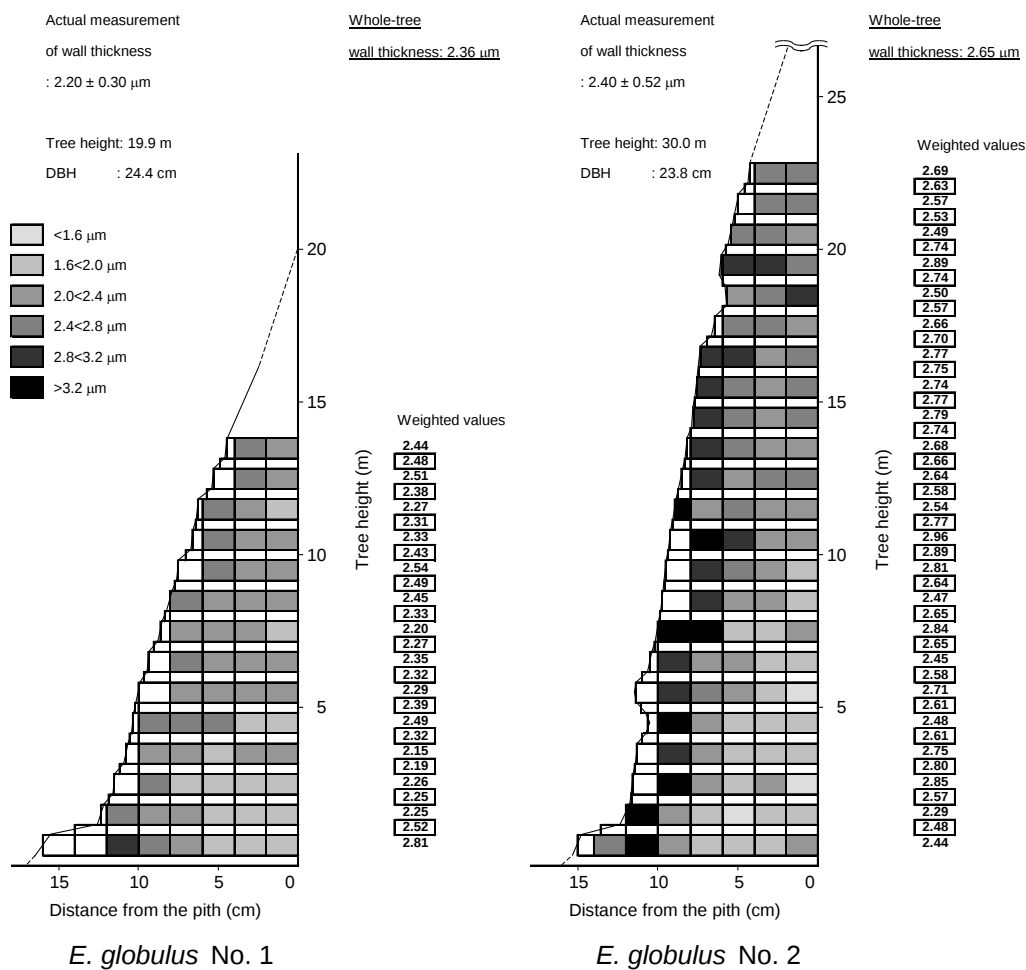
図 20 E. globulus における繊維壁厚の樹幹内変異
