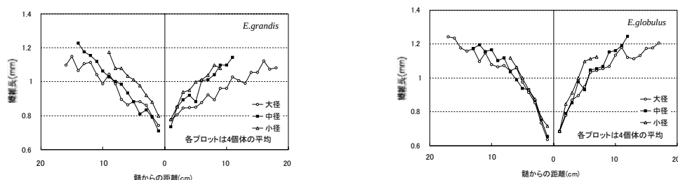
図 37 ユーカリ類の繊維長の半径方向分布
