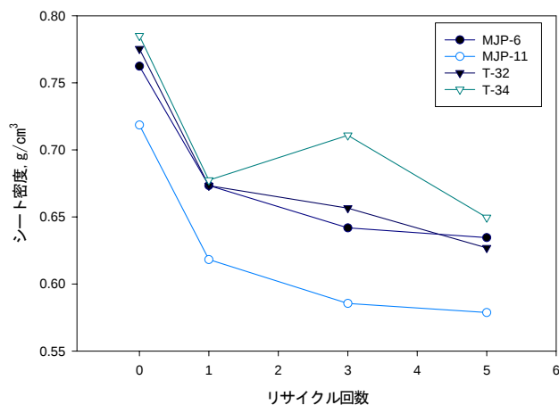
図3 リサイクル回数とシート密度
