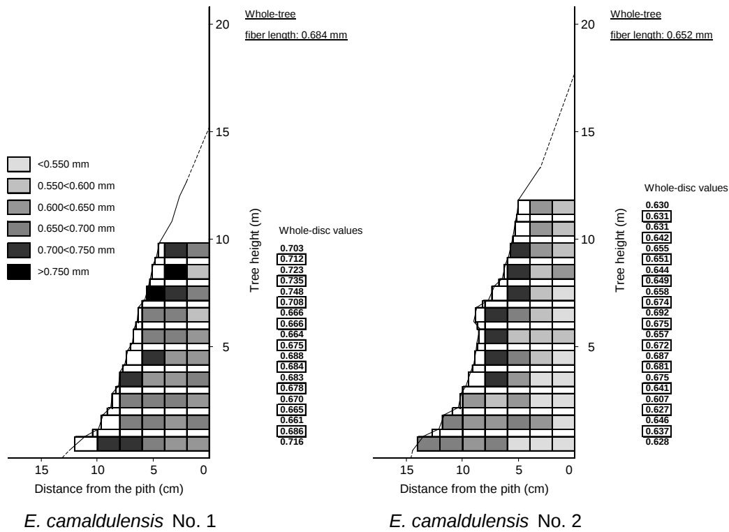
図 17 E. camaldulensis における繊維長の樹幹内変異
