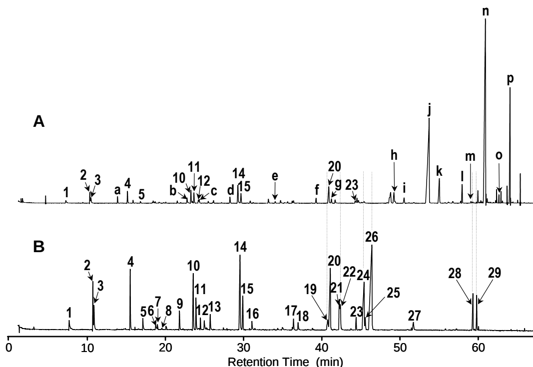
図 25 アセチル化後(A)とアセチル化前(B)のクロマトグラム
