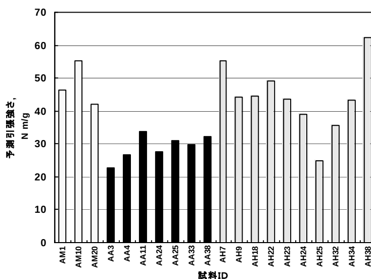
図5 比引張強さの予測収束値
