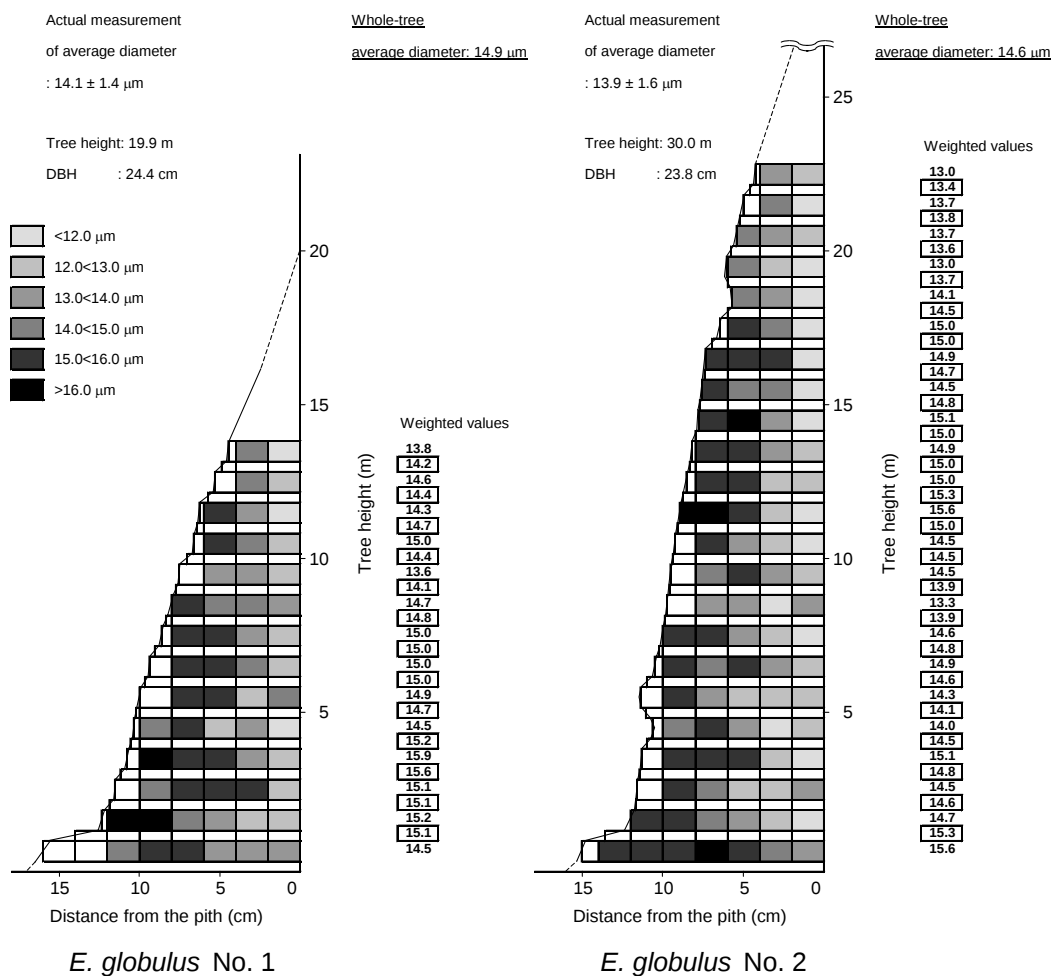
図 22 E. globulus における繊維直径の樹幹内変異
