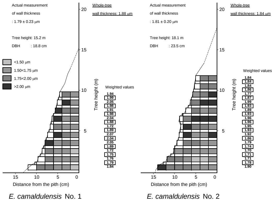
図 19 E. camaldulensis における繊維壁厚の樹幹内変異
